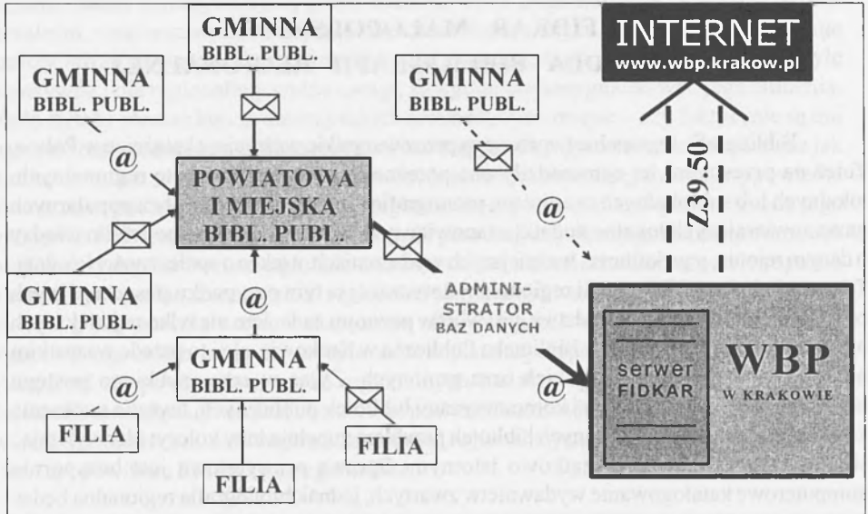
Rys. 1. Schemat funkcjonowania katalogu centralnego dla bibliotek małopolskich
